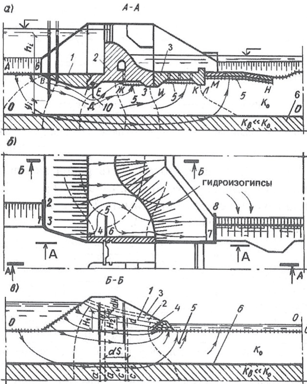
Рисунок П.2.4– Схема фильтрации воды:
