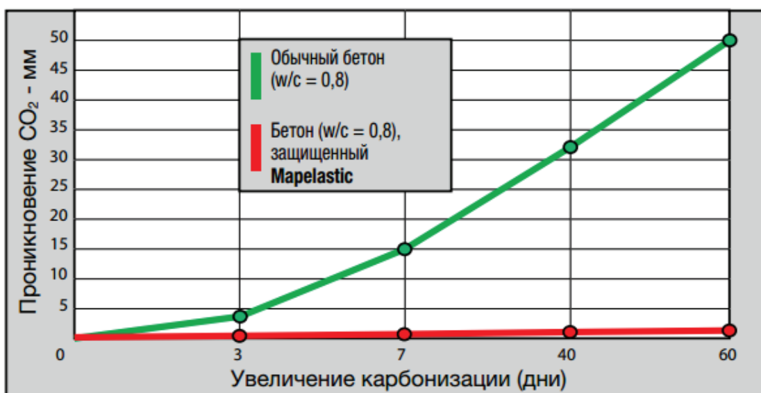
Рис.12.2 – Защита Mapelastic пористого бетона от ускоренной карбонизации (30% CO 2 )
