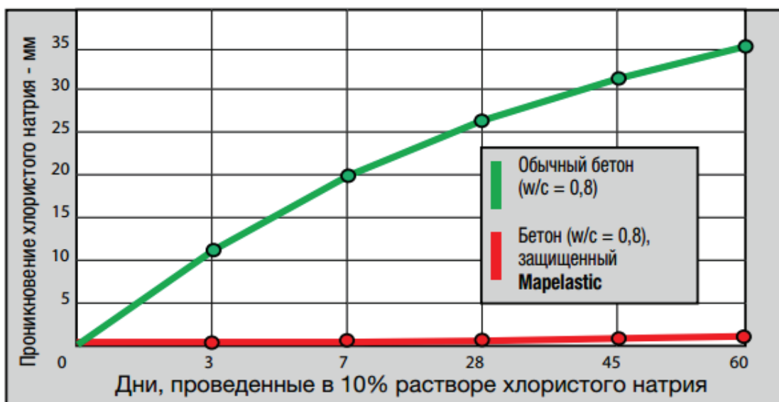
Рис. 12.3 – Защита Mapelastic пористого бетона от проникновения хлористого натрия Рисунок 12.4 показывает снижение механической стойкости (начальная 65 Н/мм 2 ) бетона, постоянно погруженного в 30% раствор CaCl 2 . В этом случае Mapelastic также эффективно защищает бетон и предотвращает агрессивное и разрушающее действие солей на бетон.
