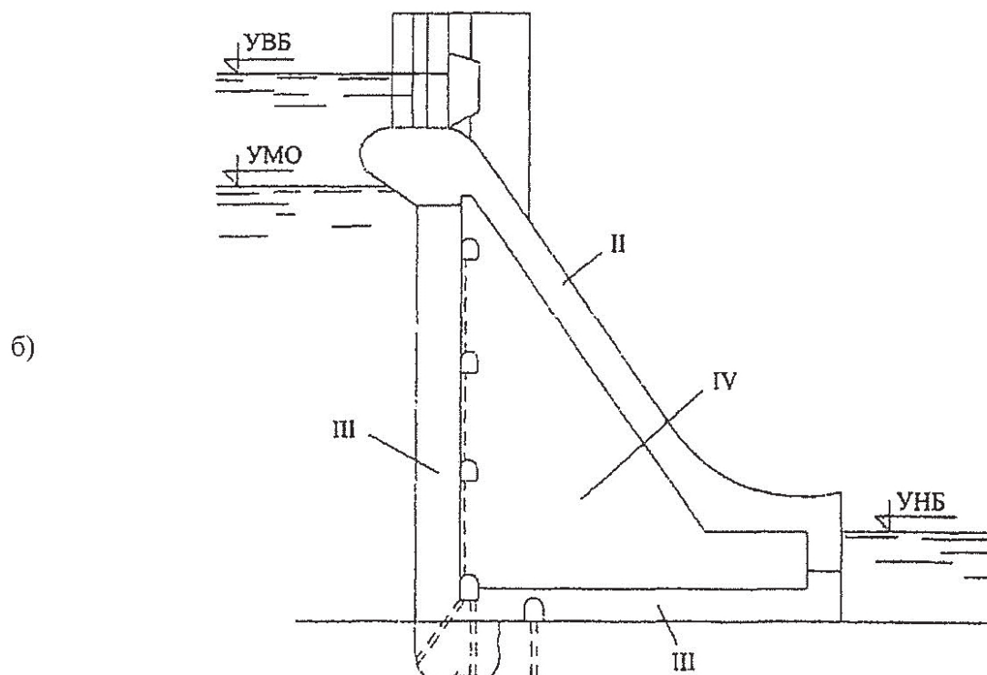
Рисунок П.3.1 – Распределение бетона в теле плотины по зонам а) – глухая плотина; б) – водосливная плотина; I-IV- зоны плотины
